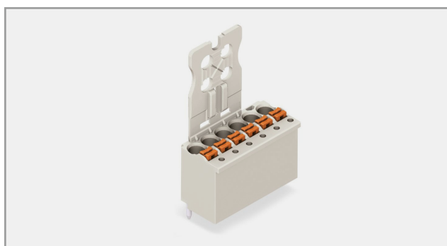
System wielowtyków picoMAX®
